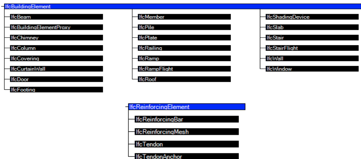
Рисунок 1 "Схема для формата IFC2x3 и IFC4"
